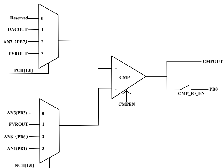
图 13.3 比较器结构图
