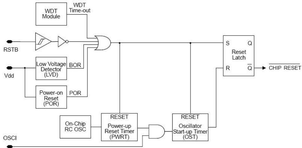
图 4.3 电路结构图
