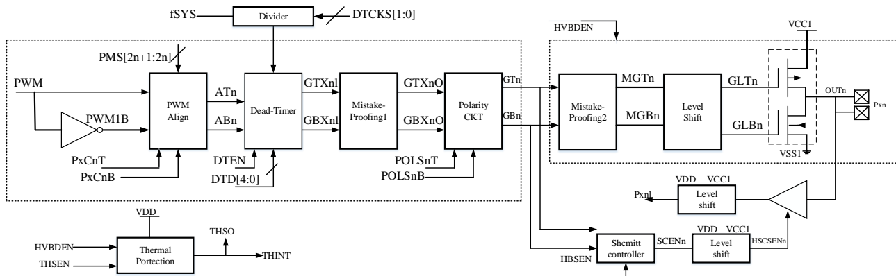
H-Bridge 驱动器结构图（n=0 代表 H 桥左臂，n=1 代表 H 桥右臂）
