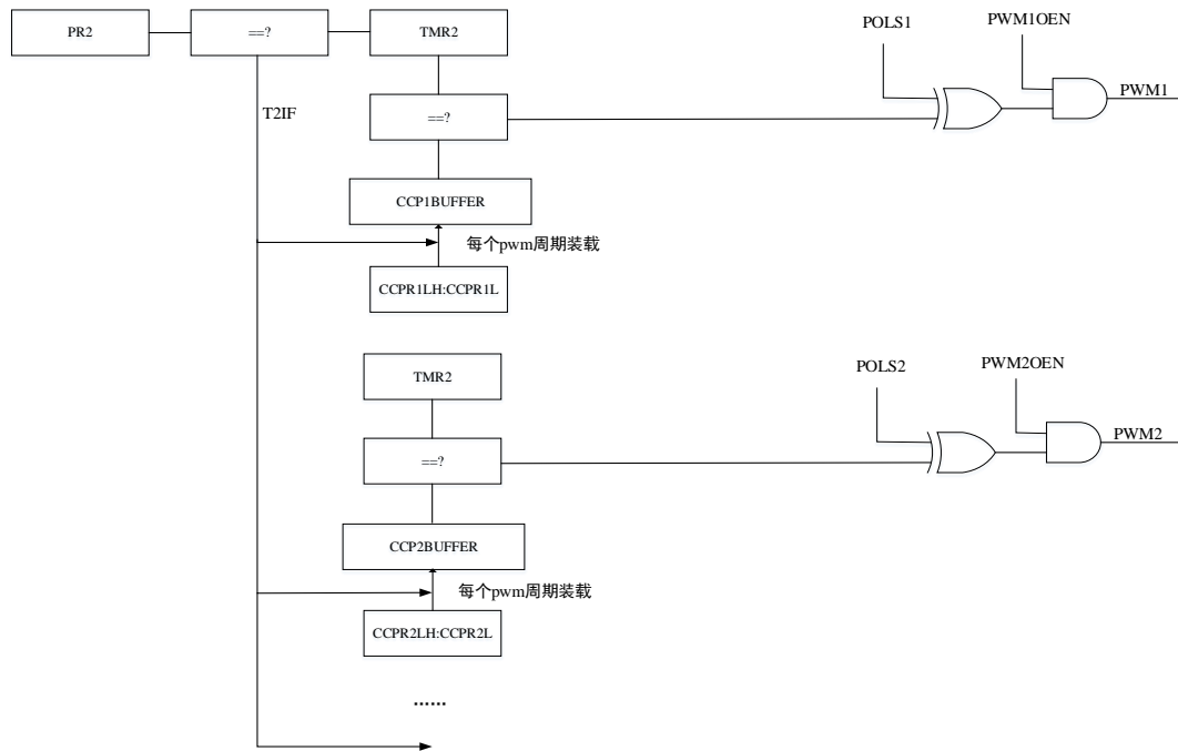
图 8.4 PWM 模块的简化框图
