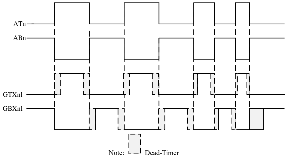
死区时间方框图（n=0 代表 H 桥左臂，n=1 代表 H 桥右臂）
