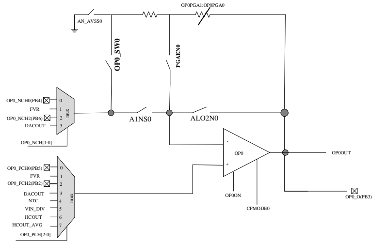
图 13.1 运放 OP0 结构图
