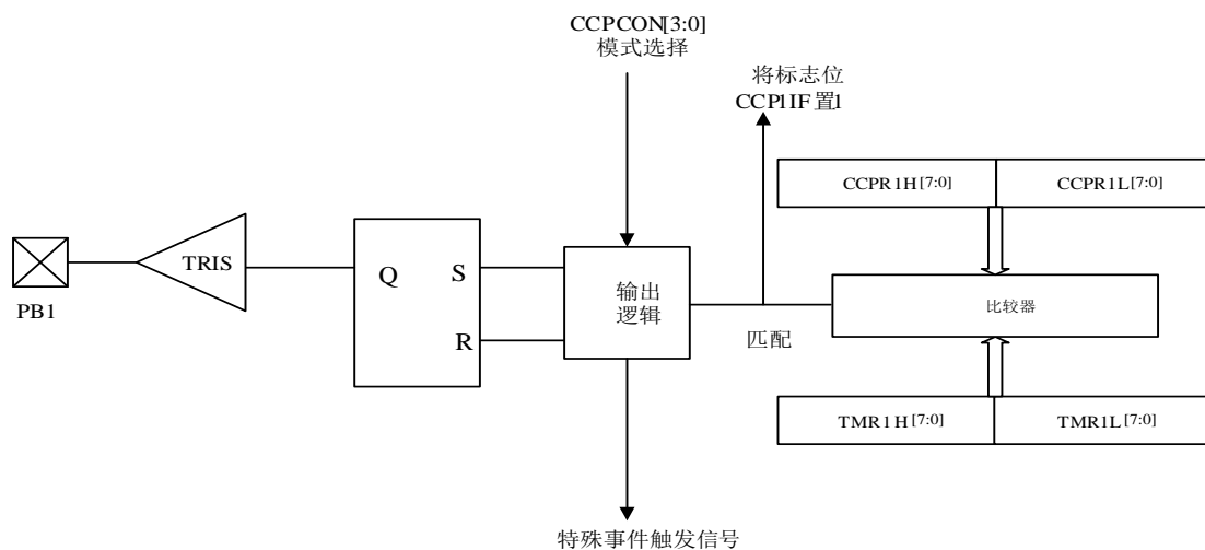
图 8.3 比较模式工作原理图
