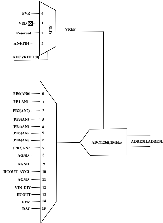
图 14.1 A/D 结构图
