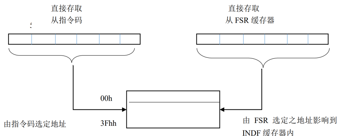
图 2.1 直接/间接存取
