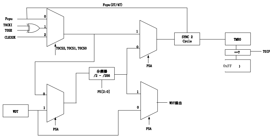
图 7.1.5: Timer0/WDT Prescaler 结构图
