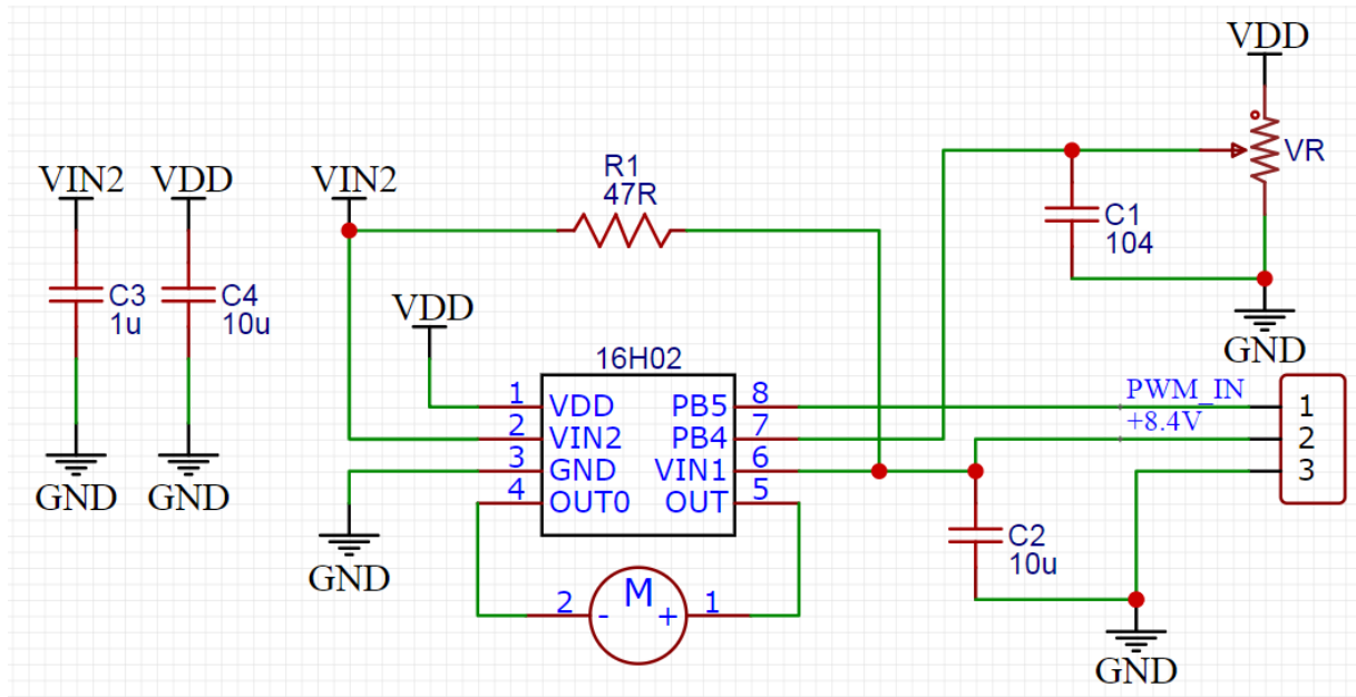
AD16H02 典型电路应用
