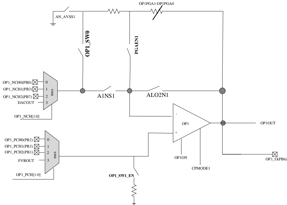
图 13.2 运放 OP1 结构图
