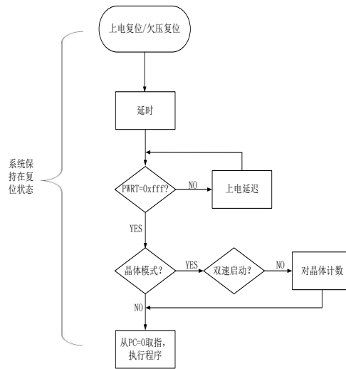
上电复位流程图
