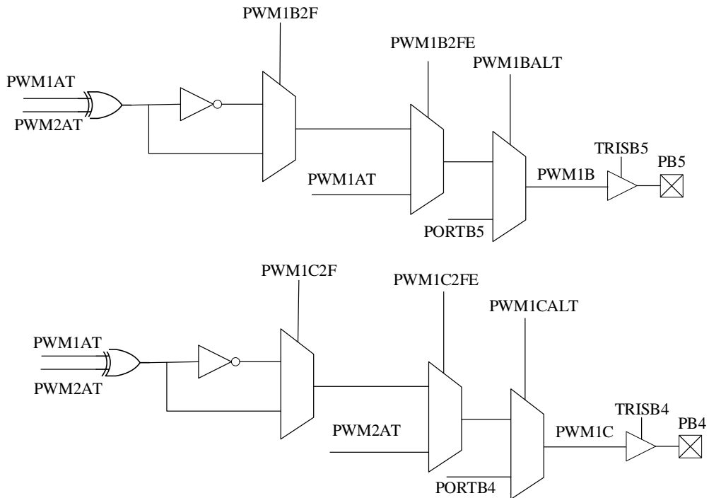
PWM 结构图 2
