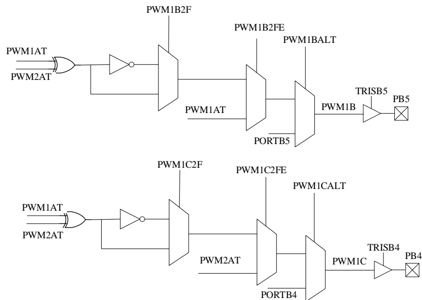
第 2 功能功能输出结构图
