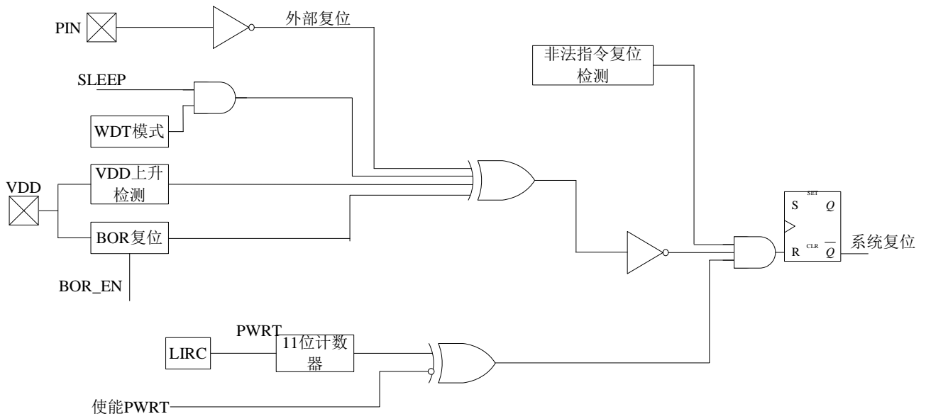
复位框图
