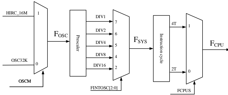
时钟原理图
