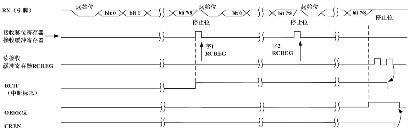
UART 接收原理图
