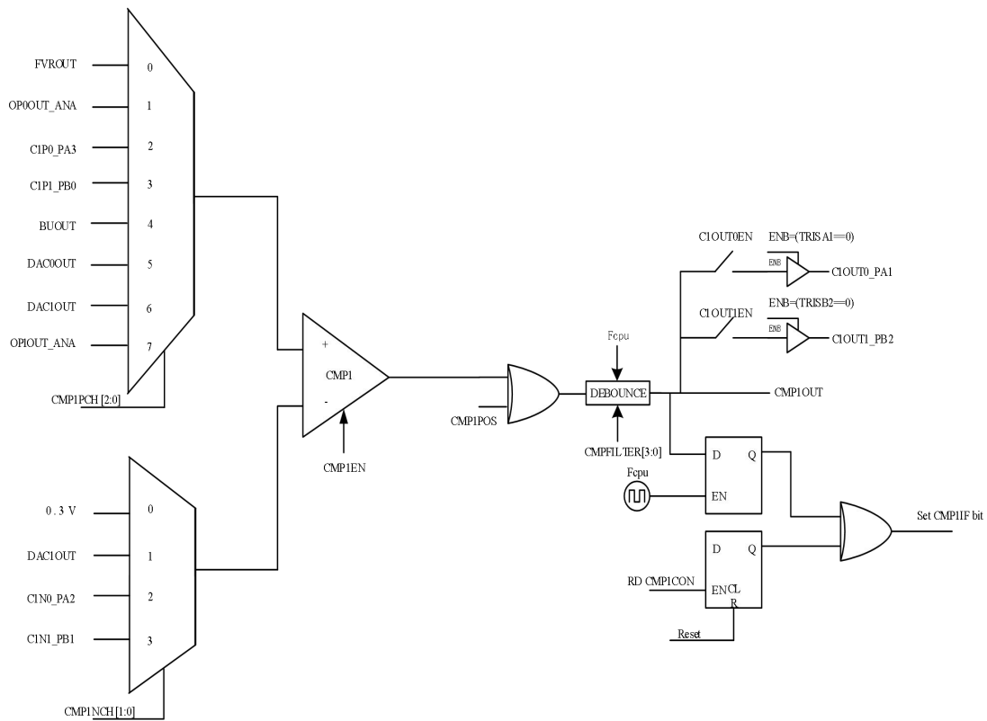
CMP1 电路图
