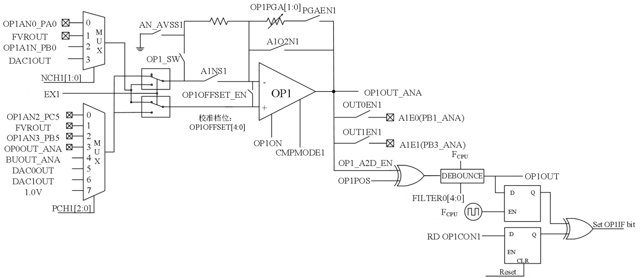
OP1 电路图
