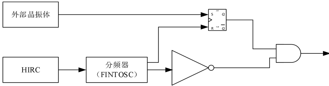
FSCM 原理图
