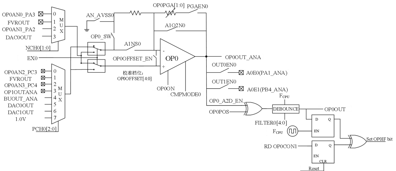
OP0 电路图
