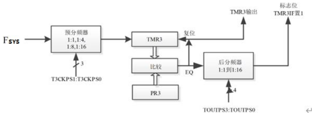
T3 结构图
