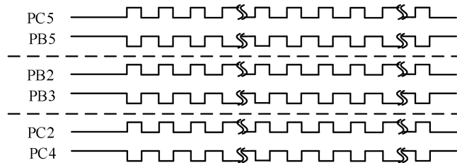
3 组 PWM 输出
