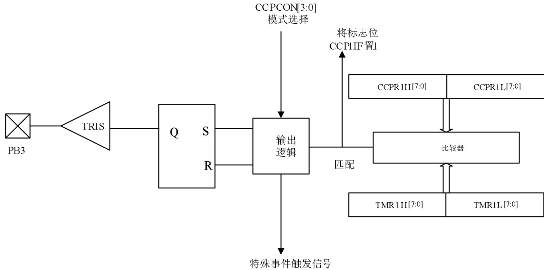
比较模式工作原理图
