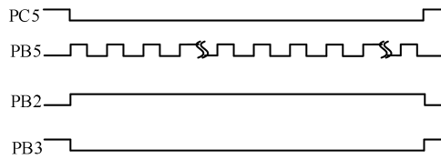
全桥 PWM 输出示例 b
