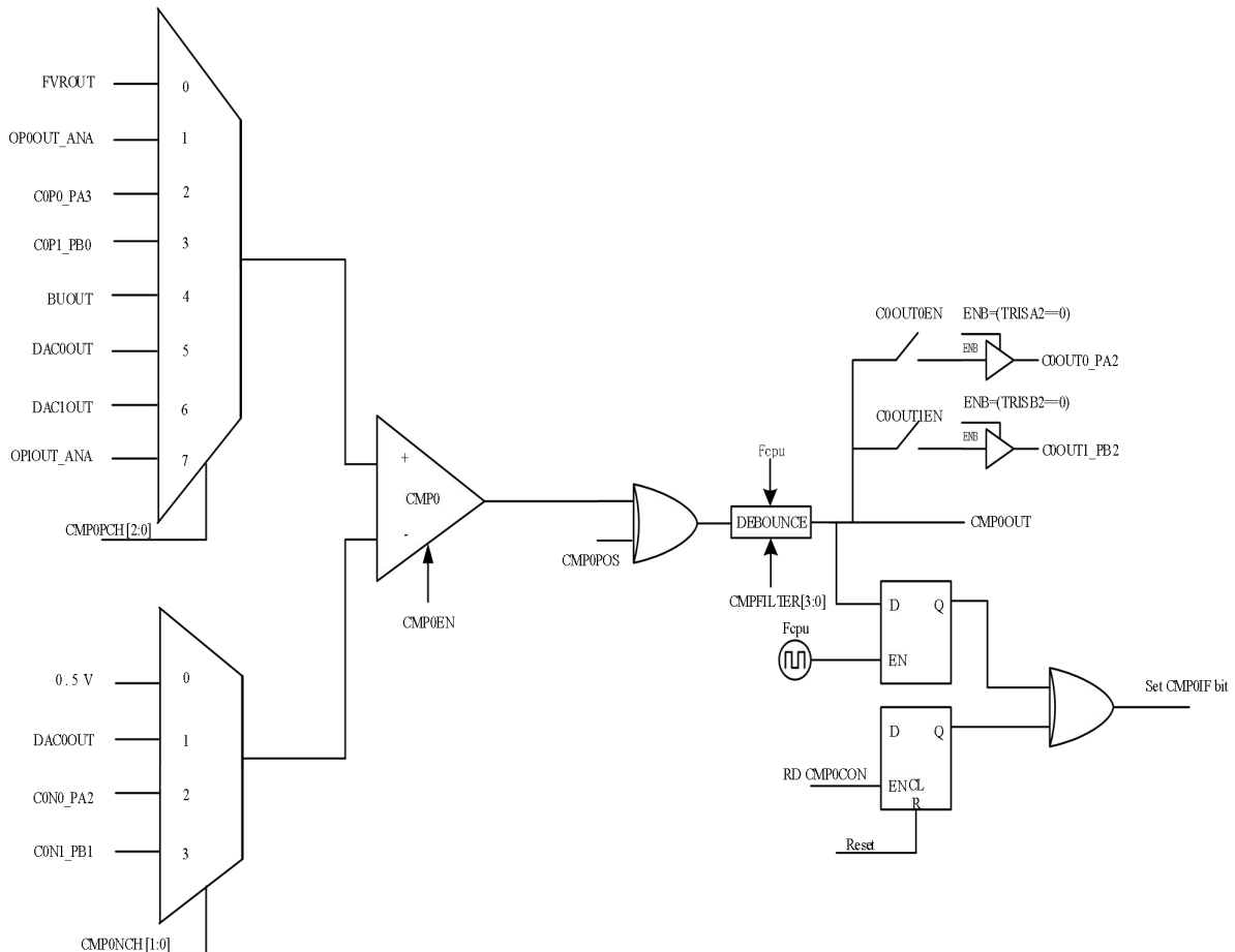
CMP0 电路图
